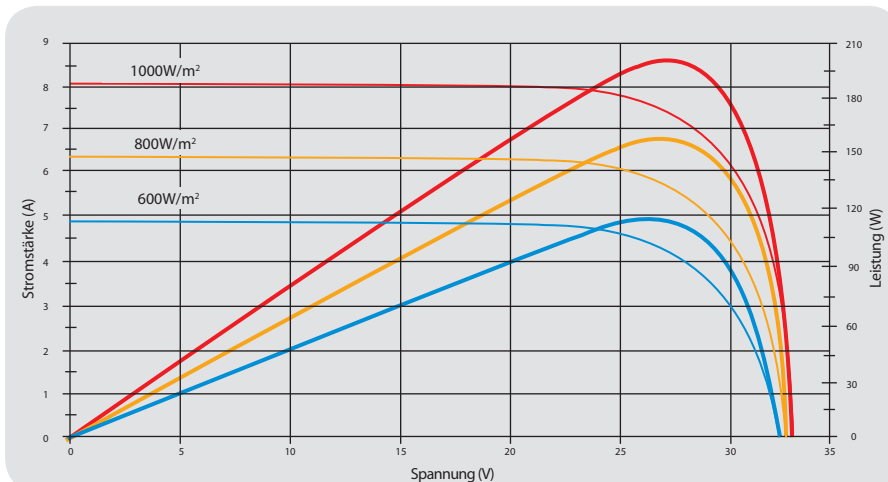
Strom-Spannungs - und Leistung-Spannungskennlinie (200W)
